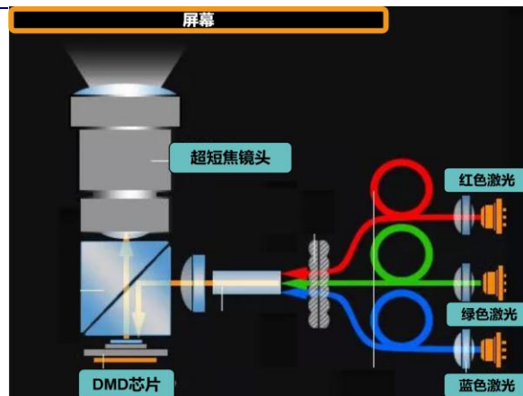
图 27：激光电视结构图
