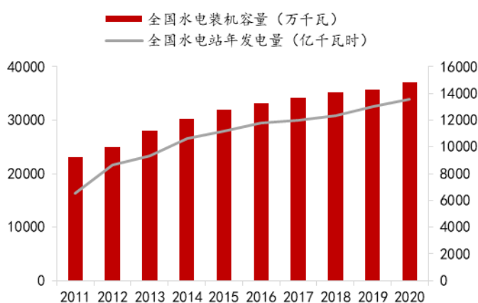
图1： 全国水电站装机容量与发电量
