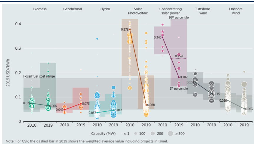
图 30：光伏进入平价时代，全球渗透率享 10 倍空间
