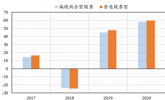
图37: 基金收益率连续两年稳步走高(单位: %)
