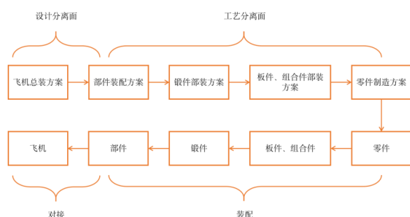
图 12：飞机制造方案：零件-组合件-锻件-部件-整机
