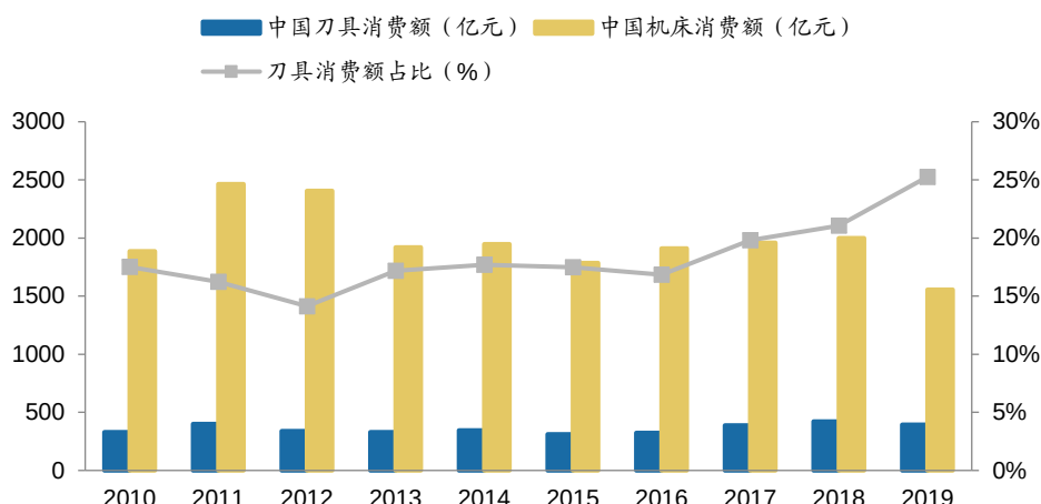
图 20: 中国机床和刀具消费额
