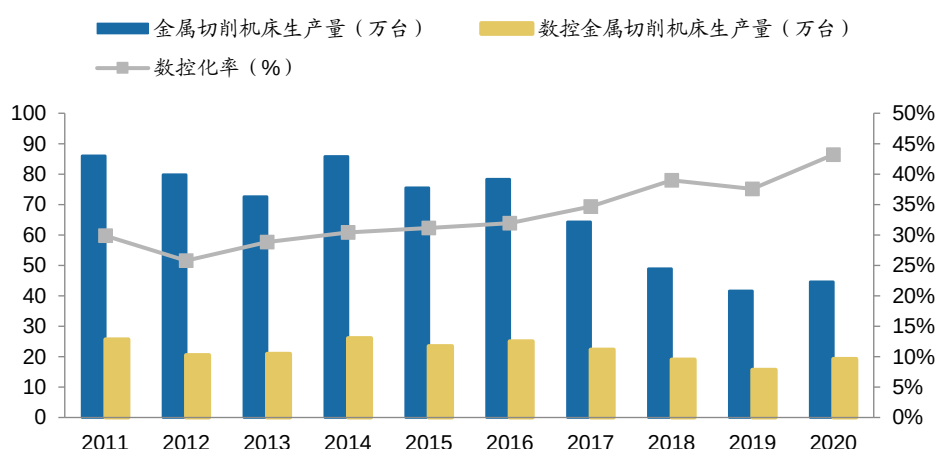
图 21: 中国金属切削机床产量和数控化率
