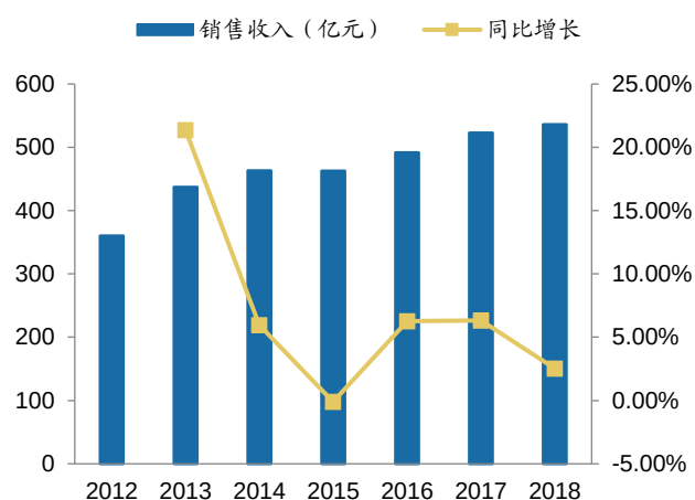
图 10: 2012-2018年中国空气压缩机行业销售收入
