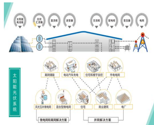
图 45：太阳能光伏系统示意图
