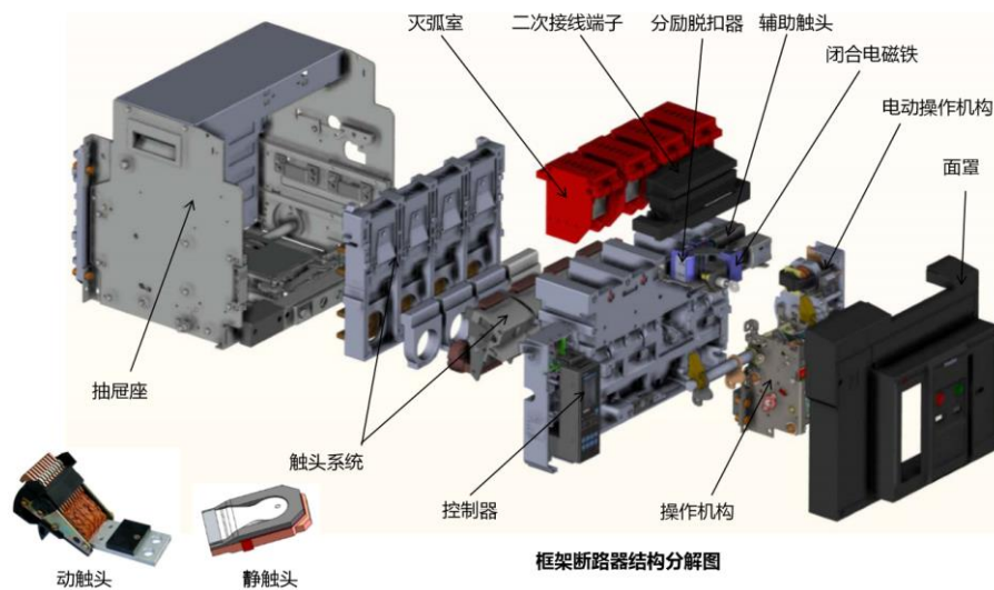
图 20：低压电器产品多为机械+电磁结构（智能低压电器含通讯模块等新增部件）
