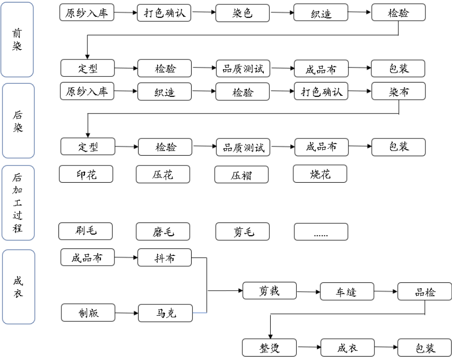
图41、制衣工艺流程图
