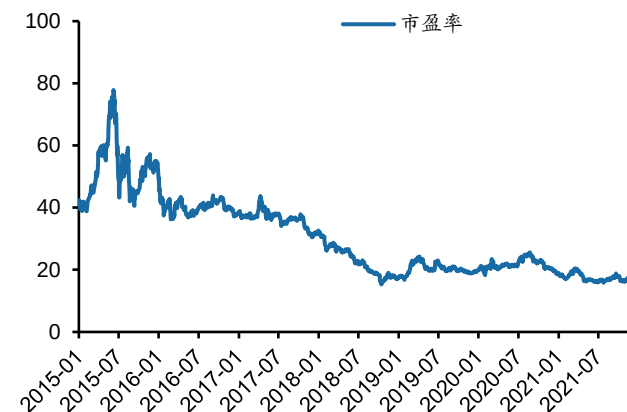
图 7：板块估值位于历史底部
