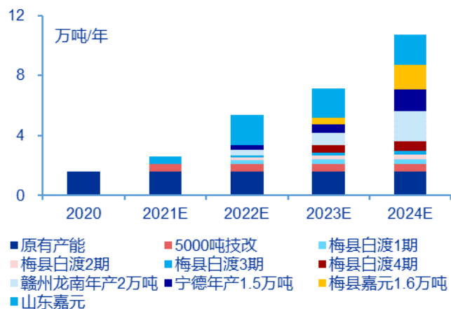
预计2023年嘉元科技铜箔总产能达7.2万吨
