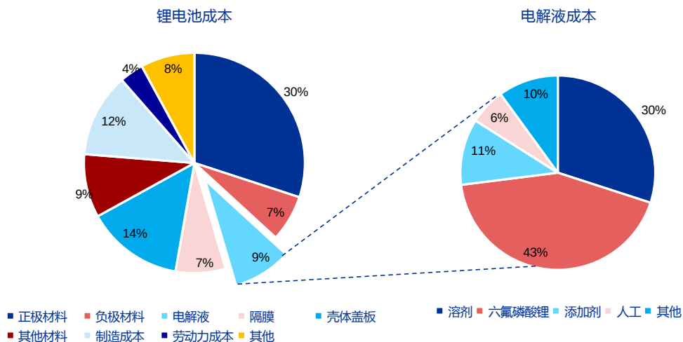
电解液原材料成本占比超80%
