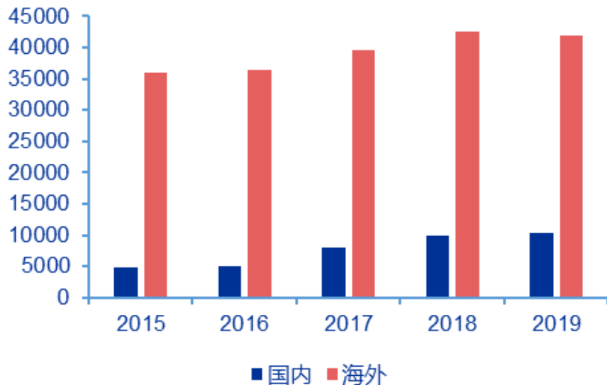
全球电炉钢产量（万吨）
