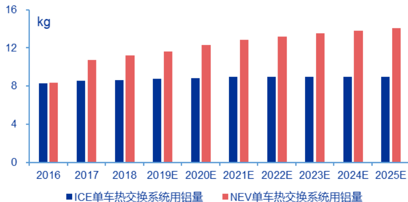
2016-2025年中国纯电动车和燃油车热交换系统单车用铝量
