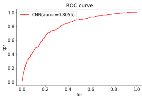
图 9: CNN 模型的 ROC 曲线图
