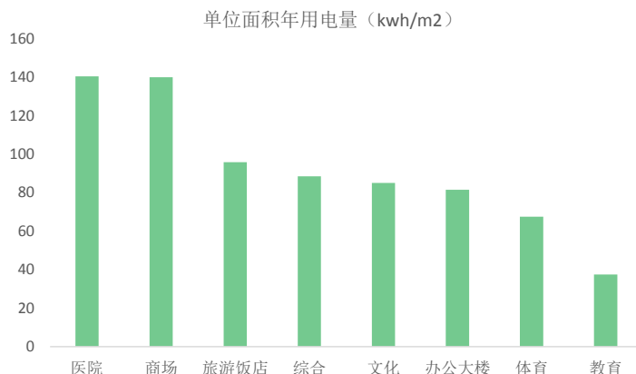
图 21：2020 年上海市各类型公共建筑年用电强度，医院商业名列前茅
