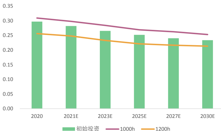
图 19：2030 年 1000h 发电小时地区分布式光伏 LCOE 有望下降超 15% （元）
