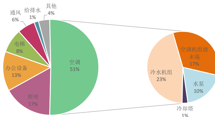
图 27：典型商业建筑能耗 75%来自空调、照明、通风、给排水领域
