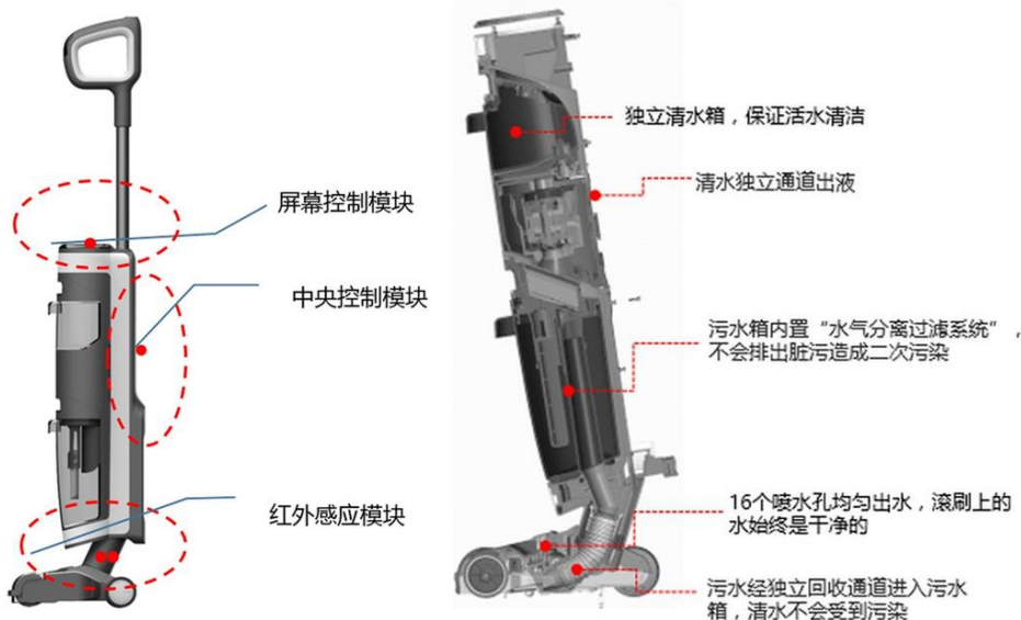
图 13：芙万洗地机产品细节图及工作原理
