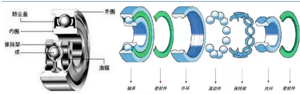
图表21： 轴承内零部件示意图
