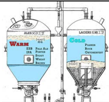
图表3：拉格工艺与爱尔工艺
