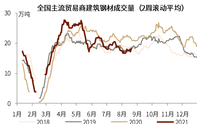
图表 19：建筑钢材成交量周环比回升
