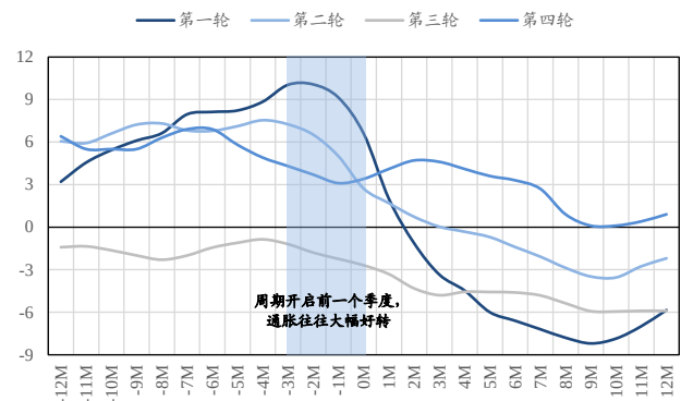
图 4: 特征二: 通胀快速回落
