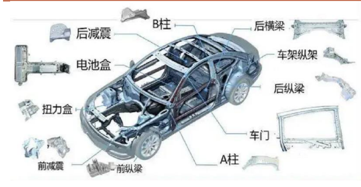
图 14：冲压零部件在车身上应用
