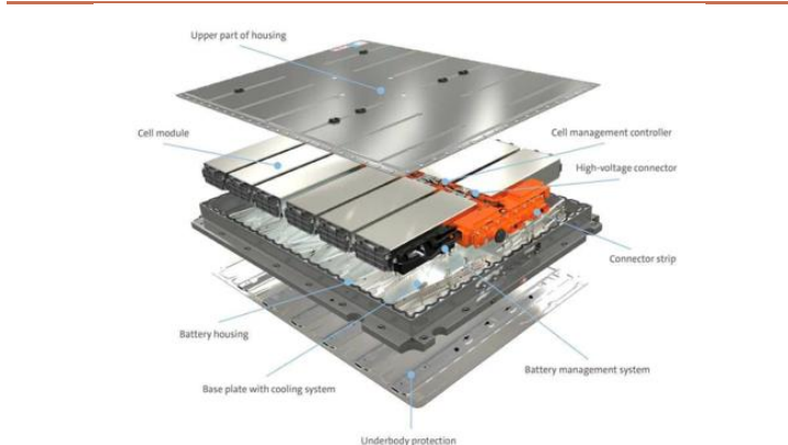
图 16：新能源汽车电池系统
