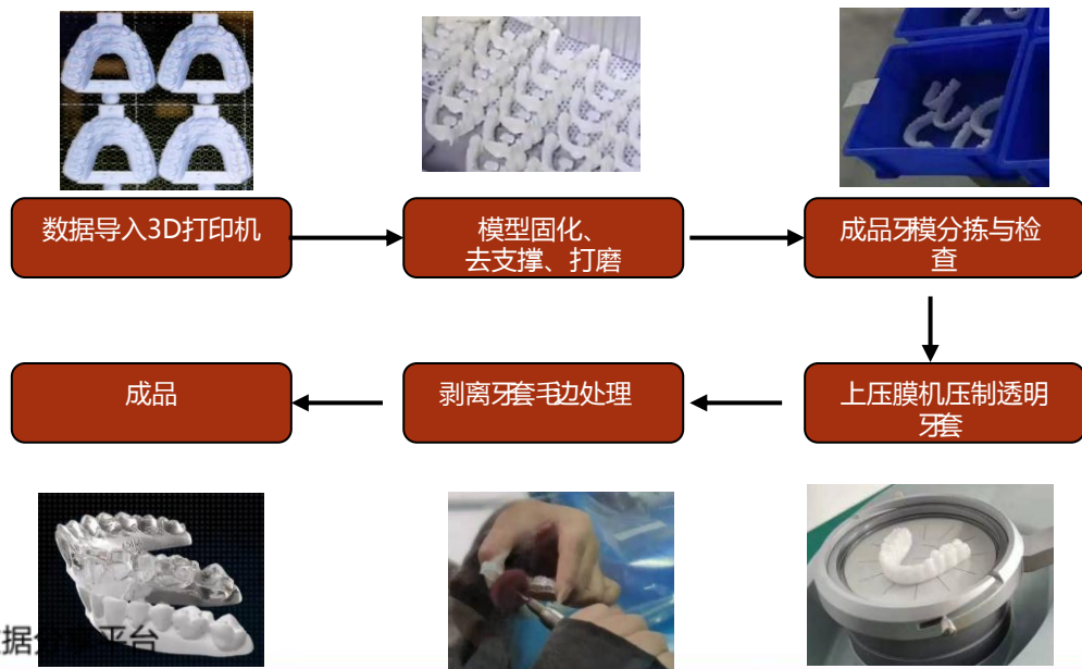
图表12 隐形牙套 3D打印加工过程
