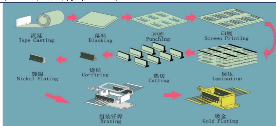
图 73、电子陶瓷外壳生产工艺流程
