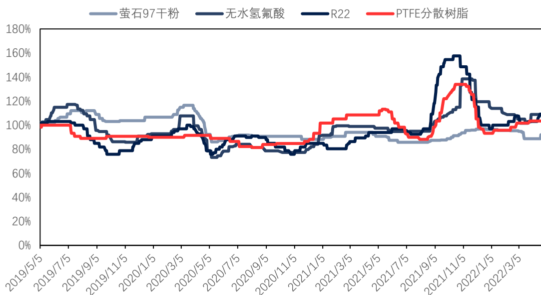
图 10：氟化工价格近 3 年的变动趋势
