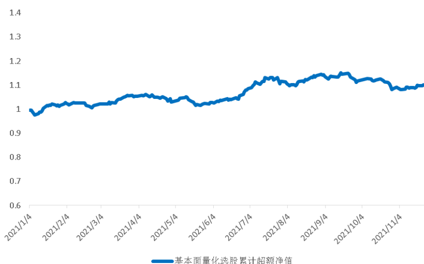
图 3 基本面因子量化选股模拟净值
