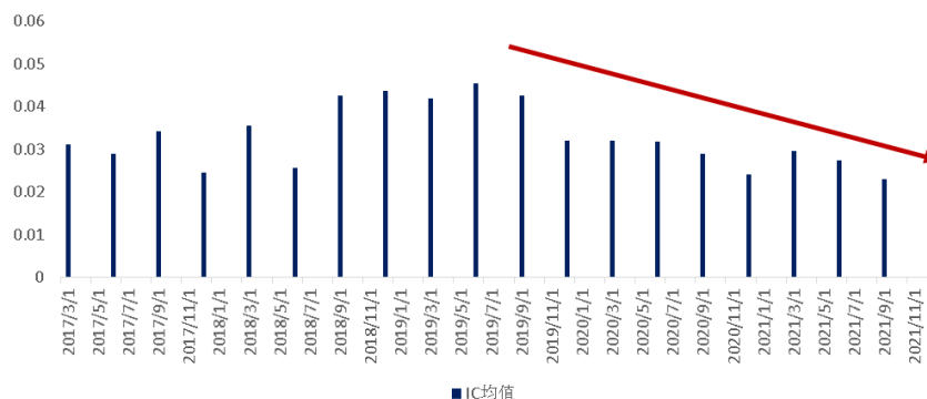
图 2 公开量价因子平均日度 IC
