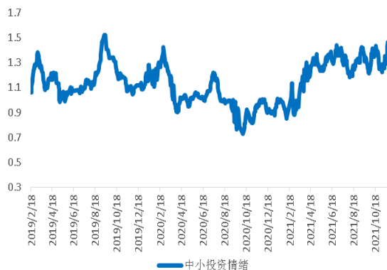
图 5 中小投资情绪指数走势
