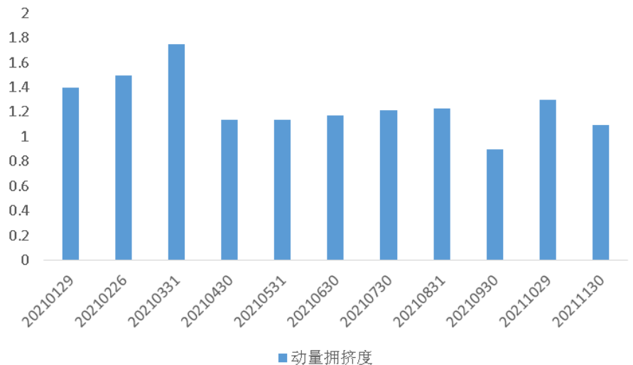
图 4 2021 年动量拥挤度指标月得分
