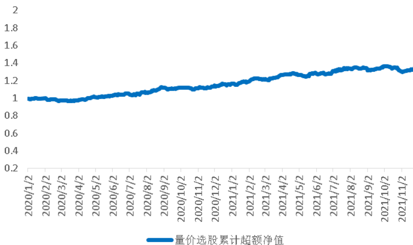
图 7 量价因子量化选股模拟净值
