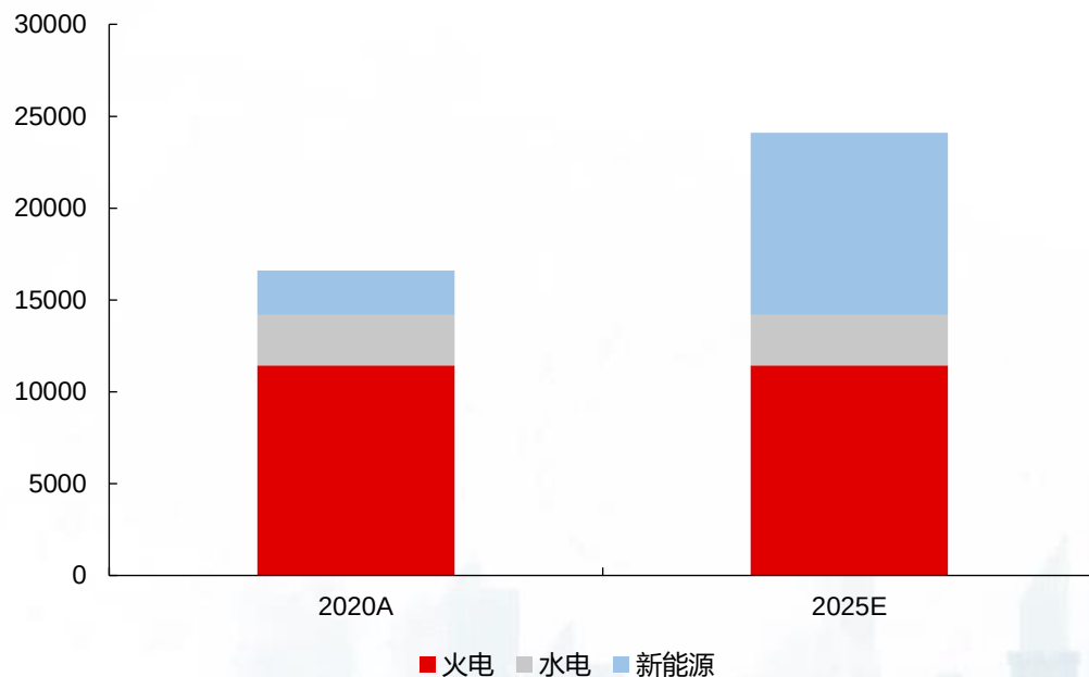
图：不考虑火电水电新增华电集团装机演变（单位：万千瓦）
