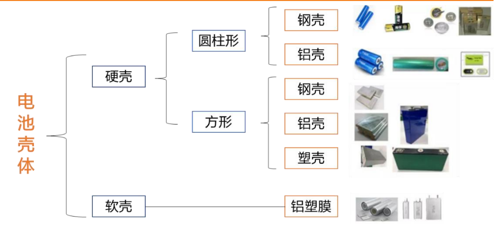
图 14：锂电池分类
