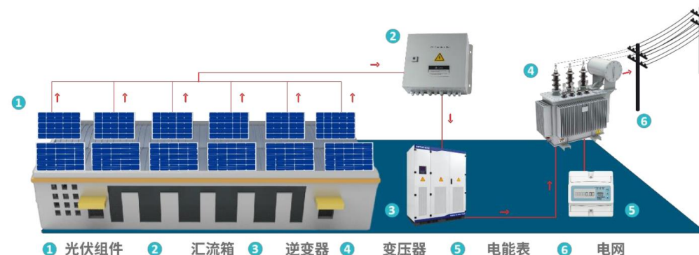
分布式光伏电站示意图
