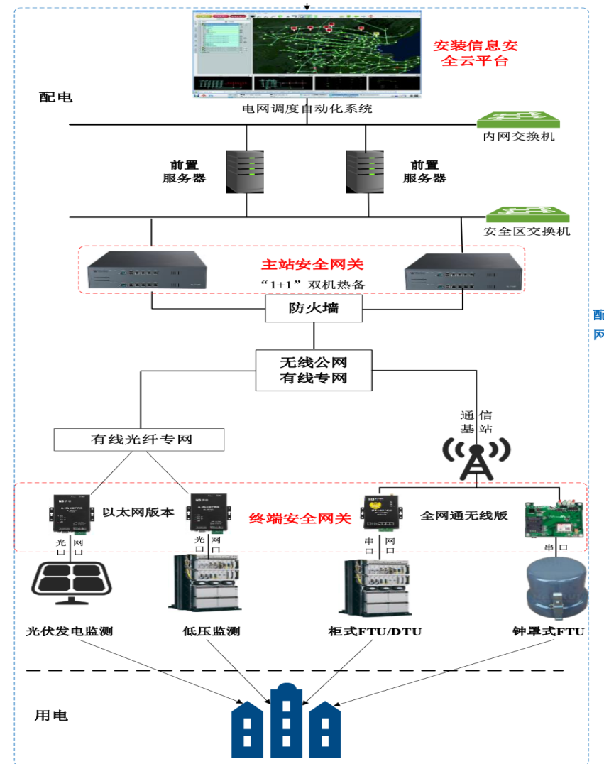
维德信息配电信息安全结构图
