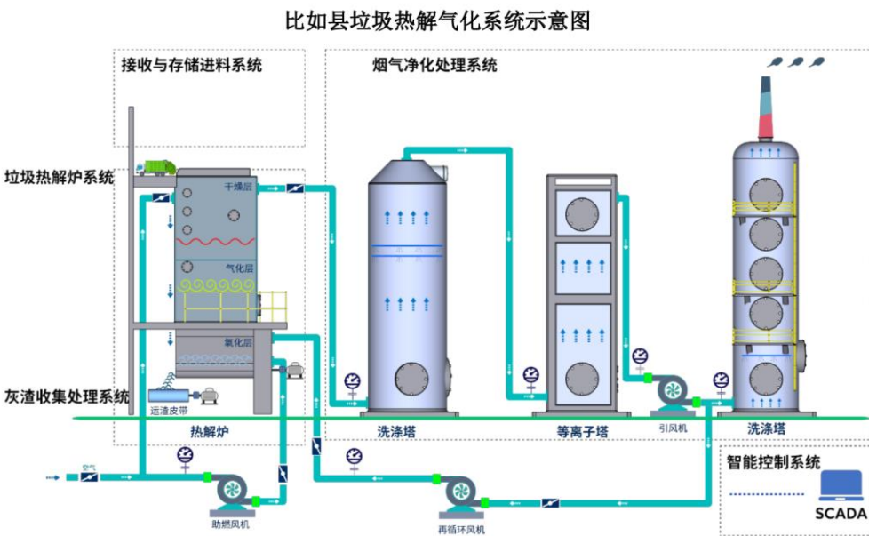
垃圾热解气化系统示意图
