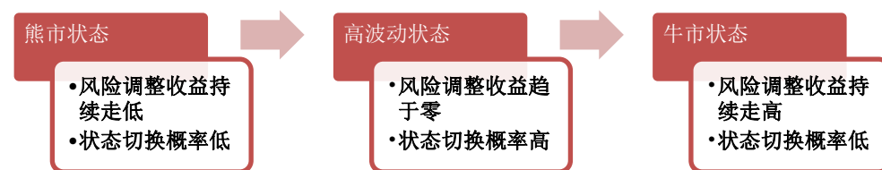
图 3：HMM 市场状态识别模型示意图
