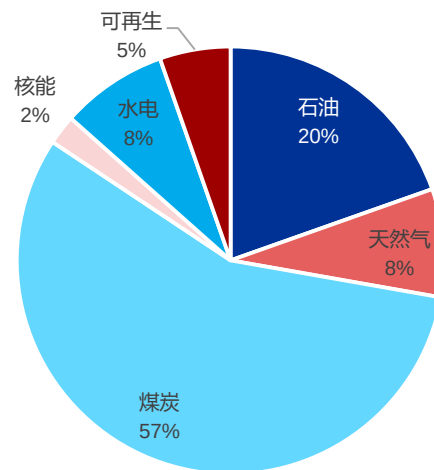
2020年中国能源消费结构占比
