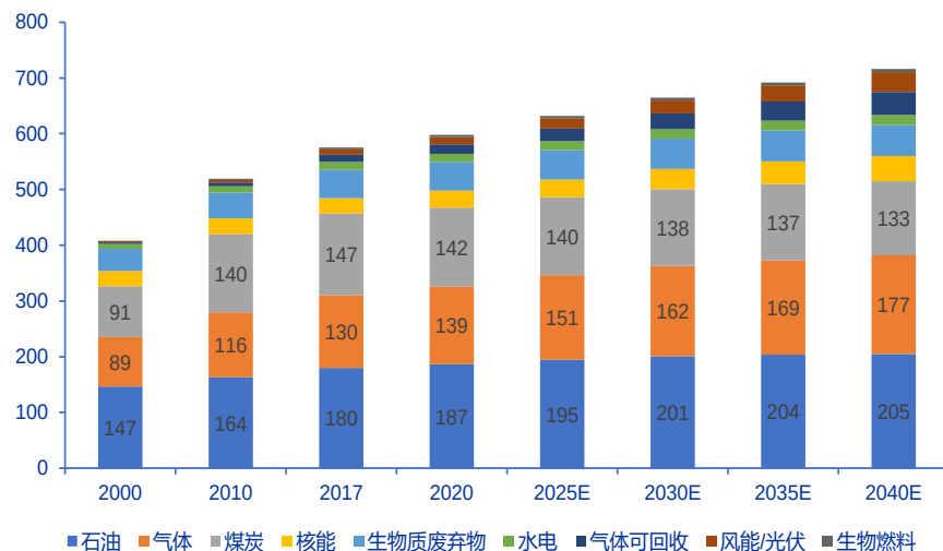
全球能源结构变化 (Quadrillion BTUs)
