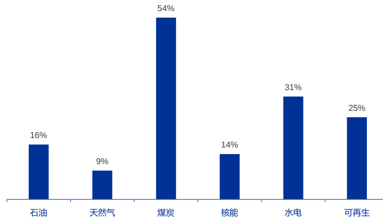
2020年我国能源消费在全球占比
