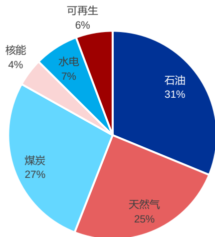
2020年全球能源消费结构占比
