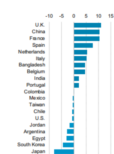
Yearly change in LNG imports, 2019
