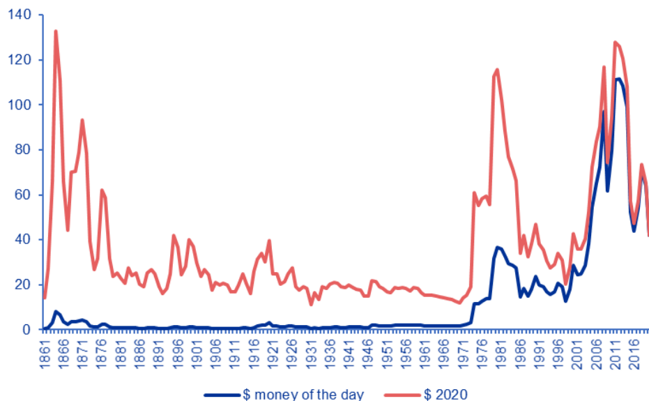
历史油价与美元调整后油价（美元/桶）
