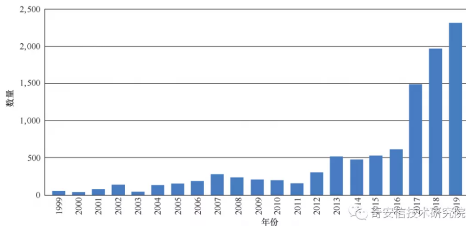
图 14: 近 20 年物联网相关 CVE 漏洞报告趋势 (1999—2019)
