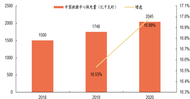
图13: 中国数据中心耗电量及增速
