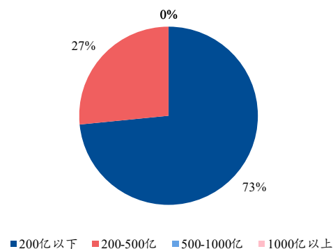
图 50、中证 500 增强 ETF_E 自由流通市值权重分布
