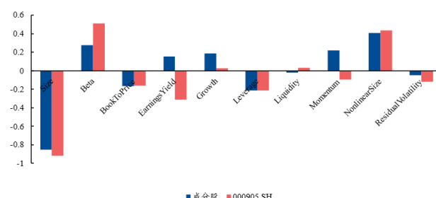
图 54、当前中证 500 增强 ETF_E 的因子暴露
