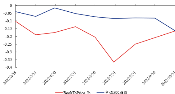
图 53、中证 500 增强 ETF_E 的 BookToPrice 暴露
