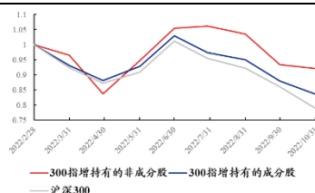
300 指增 ETF 持有的非成分股组合与 300 指增 ETF 持有的成分股组合表现
