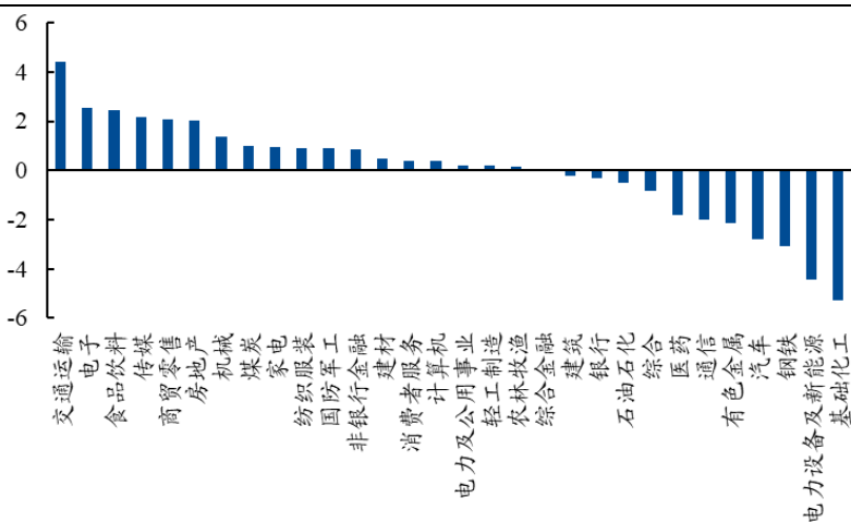
图 42、E 公司：500 增强 ETF 行业配比减去 500 增强行业配比 (%)
