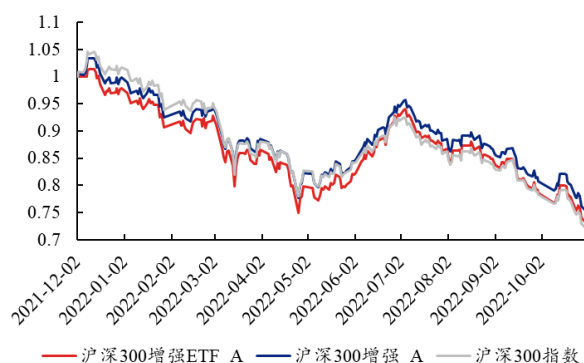
图 32、A 公司 300 增强与 300 增强 ETF
