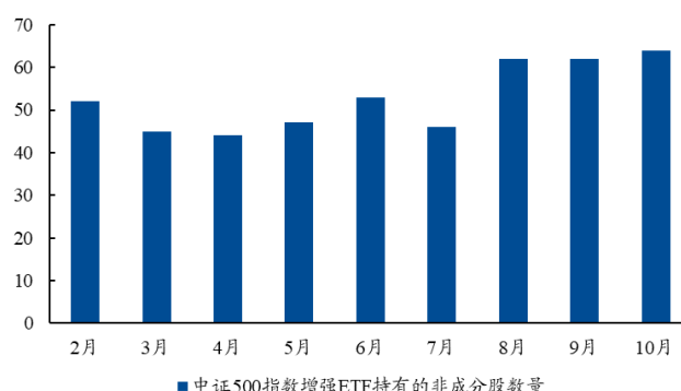
图 9、中证 500 指数增强 ETF 持有的非成分股数量 (月末统计)
