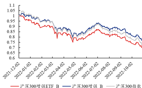
图 33、B 公司 300 增强与 300 增强 ETF
