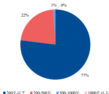
图 49、中证 500 自由流通市值权重分布
