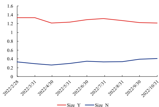
图 10、Size 暴露(被 300 指增 ETF 持有 vs 未被 300 指增 ETF 持有)
