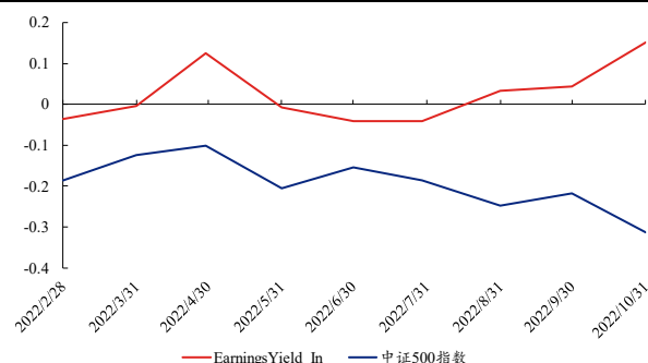
图 51、中证 500 增强 ETF_E 的 EarningsYield 暴露
