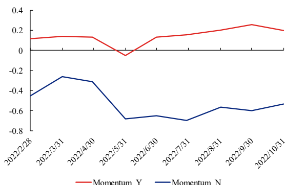
图 24、Momentum 暴露 (被 500 指增 ETF 持有 vs 未被 500 指增 ETF 持有)
