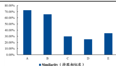
指增 ETF 与同机构同指数增强基金持股相似度
