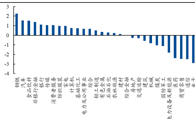
图 41、D 公司：500 增强 ETF 行业配比减去 500 增强行业配比 (%)
