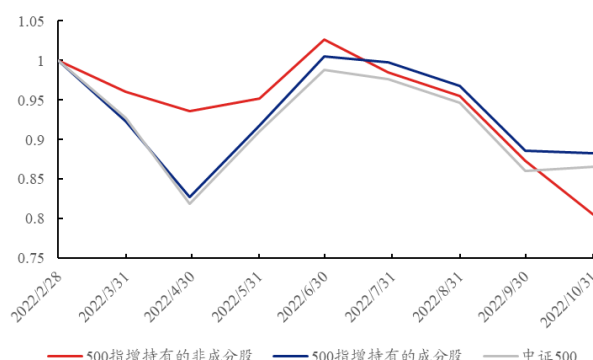
图 29、中证 500 指增 ETF 持有的非成分股组合与成分股组合表现（月末定期调仓，自由流通市值加权）
