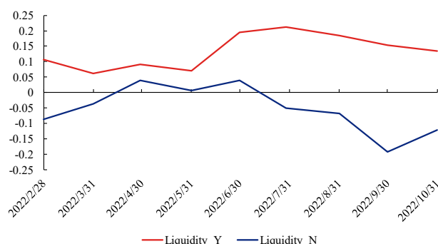
图 25、Liquidity 暴露 (被 500 指增 ETF 持有 vs 未被 500 指增 ETF 持有)
