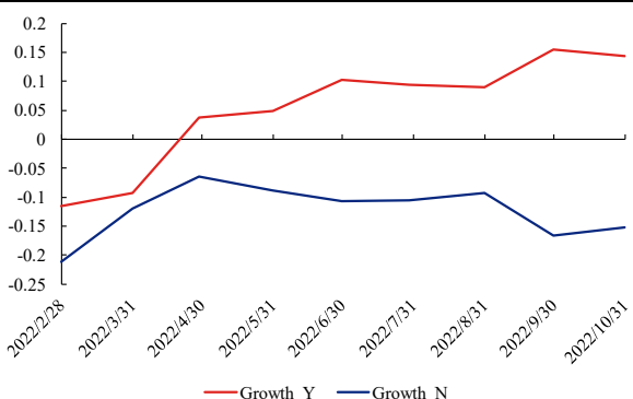
图 22、Growth 暴露(被 500 指增 ETF 持有 vs 未被 500 指增 ETF 持有)
