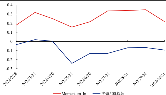
图 52、中证 500 增强 ETF_E 的 Momentum 暴露
