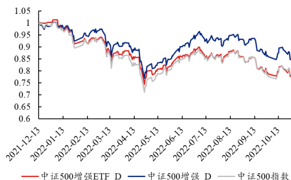
图 35、D 公司 500 增强与 500 增强 ETF
