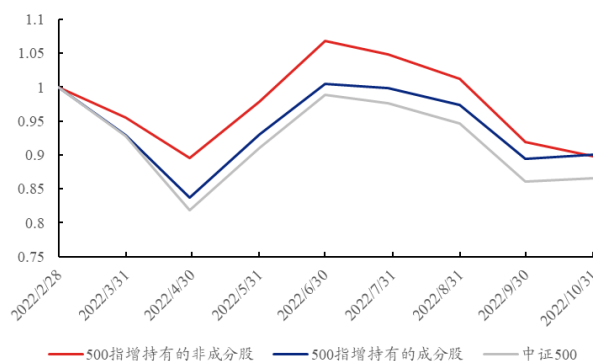
图 31、中证 500 指增 ETF 持有的非成分股组合与成分股组合表现（月末定期调仓，等权）
