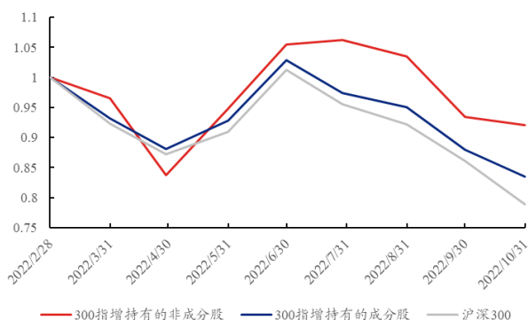
图 30、沪深 300 指增 ETF 持有的非成分股组合与成分股组合表现（月末定期调仓，等权）
