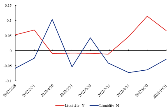
图 16、Liquidity 暴露（被 300 指增 ETF 持有 vs 未被 300 指增 ETF 持有）
