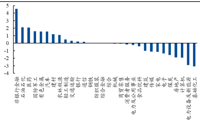
图 39、B 公司：300 增强 ETF 行业配比减去 300 增强行业配比 (%)
