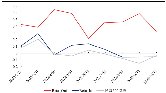
图 46、沪深 300 增强 ETF_A 的 Beta 暴露
