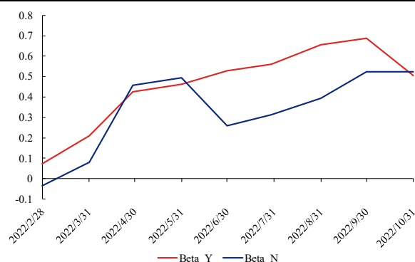
图 19、Beta 暴露(被 500 指增 ETF 持有 vs 未被 500 指增 ETF 持有)
