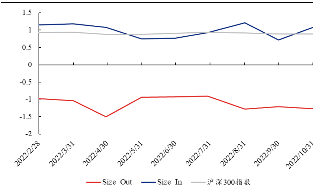
图 45、沪深 300 增强 ETF_A 的 Size 1 暴露
