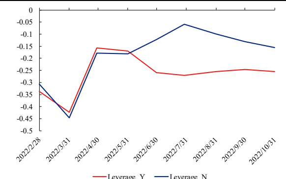
图 23、Leverage 暴露(被 500 指增 ETF 持有 vs 未被 500 指增 ETF 持有)
