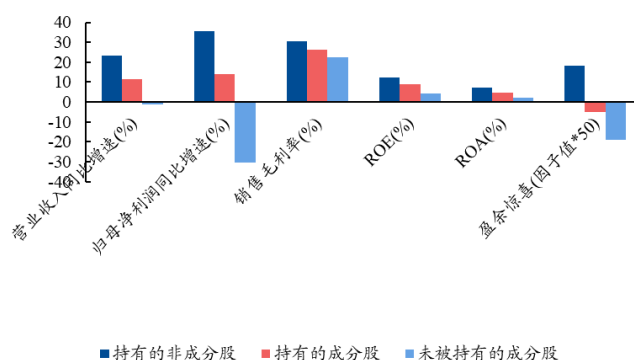
图 27、持有的非成分股 vs 持有的成分股 vs 未被持有的成分股财务数据对比 (中证 500 指增 ETF)
