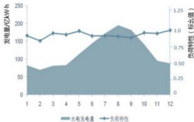
图4：云南电力负荷特性与水电出力特性对比
