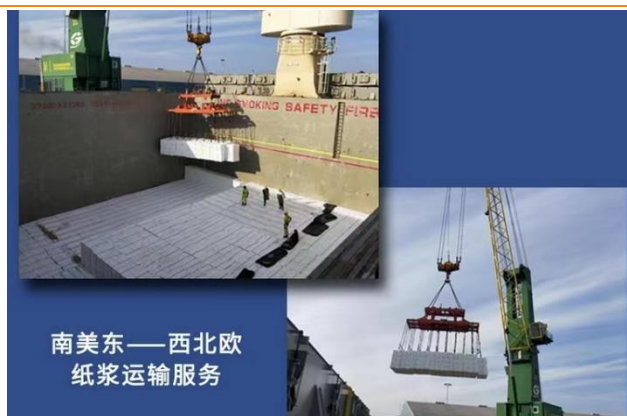
图 24: 纸浆船的船舶结构和装载纸浆的过程
