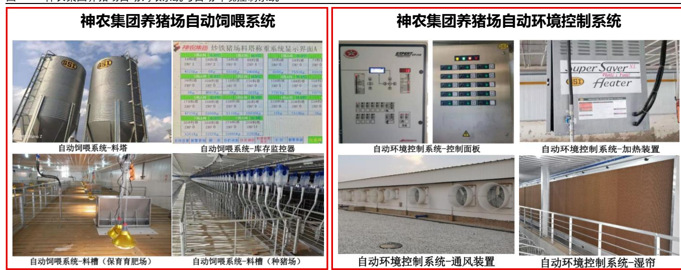
图 17：神农集团养猪场自动饲喂系统与自动环境控制系统
