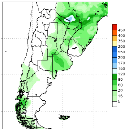
图 6：10 月 25 日-11 月 8 日阿根廷降水量（mm）
