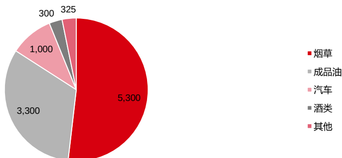
消费税结构
