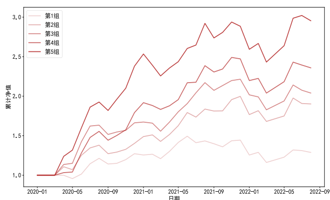
图7：基于统计期推荐成功率分组测试
