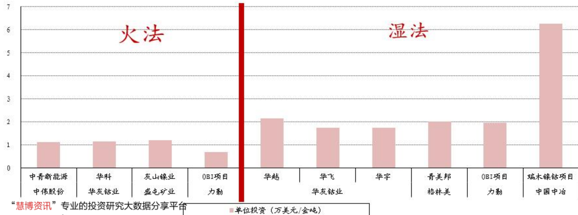
火法和湿法项目单位投资情况
