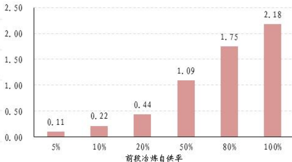
前段冶炼自供率对前驱体盈利能力影响（万元/吨）
