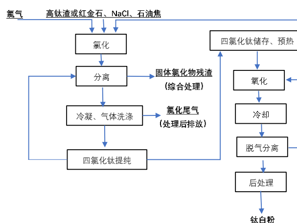
图表 29：氯化法
