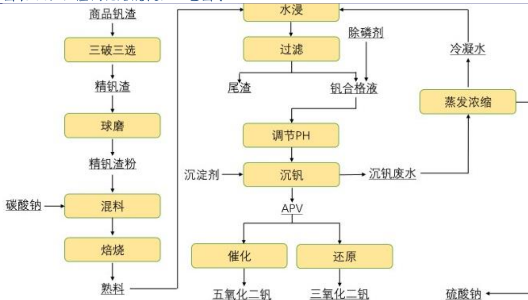
图表 14：钒渣钠化焙烧提钒工艺图示
