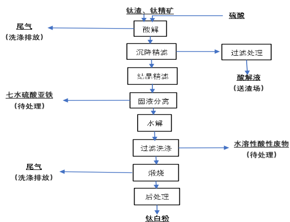
图表 28：硫酸法
