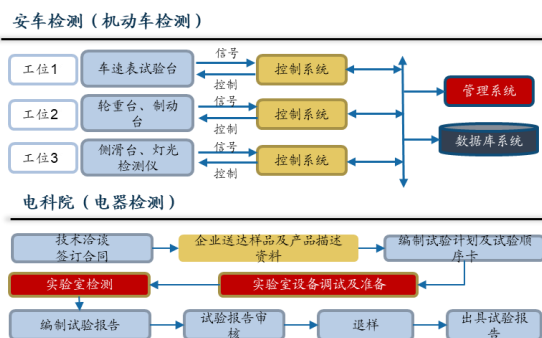
图 36：机动车检测、电器检测流程图
