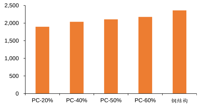
图 39：不同类型的装配式建筑建安费用（单位：元/平方米）
