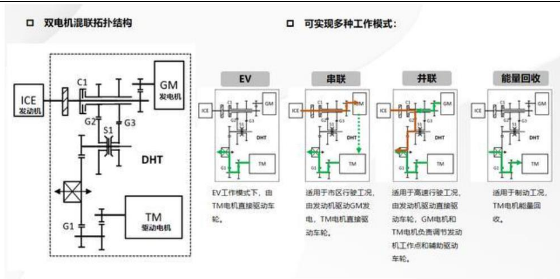
图表 21：长城汽车 DHT 拓扑结构
