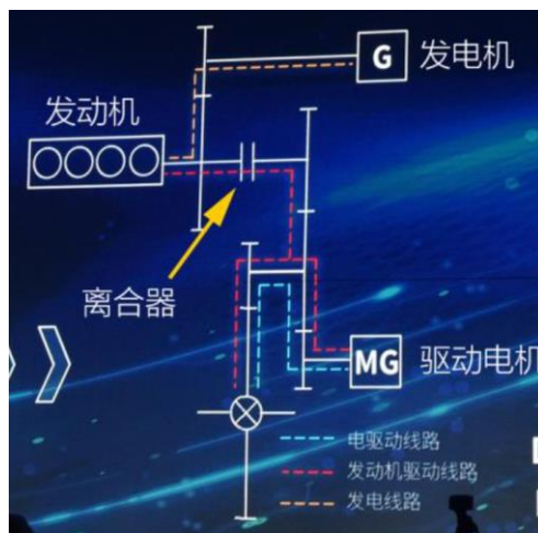
图表 20：EHS 机电耦合系统动力传递路线图
