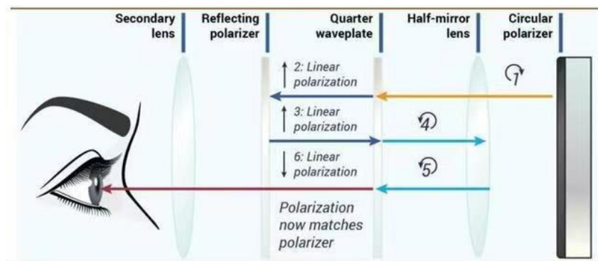
图：Pancake光学方案原理
