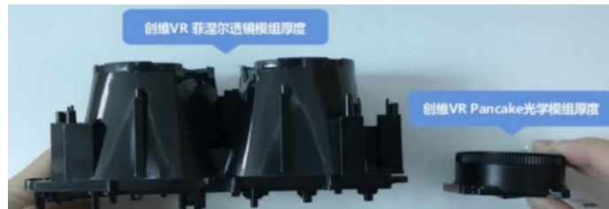
图：菲涅尔透镜模组与Pancake模组厚度比较
