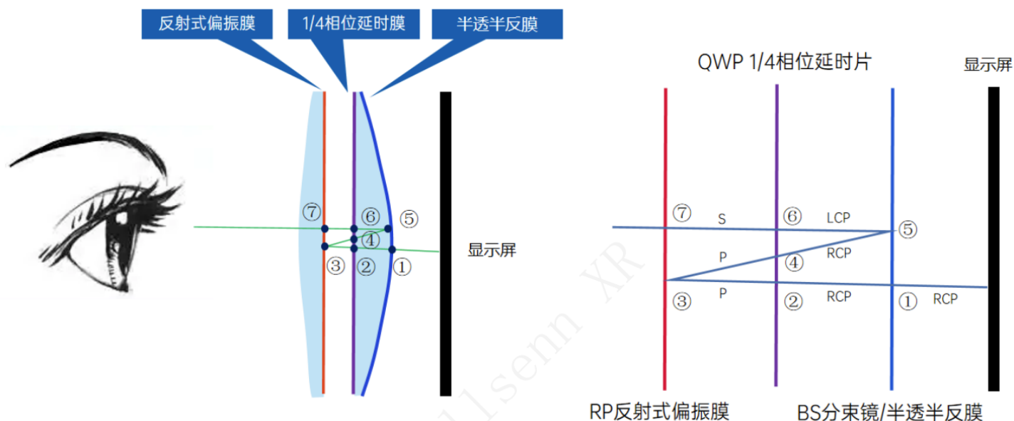
图：Pancake方案原理
