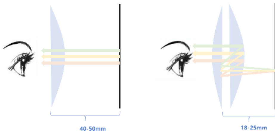
图：菲涅尔方案与Pancake方案对比
