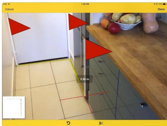
图：测量工具CamToPlan Pro操作界面
