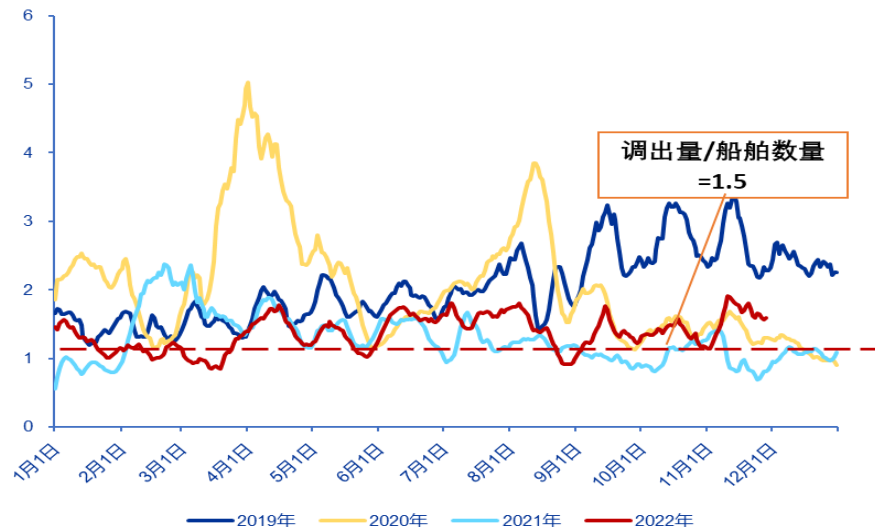
环渤海港口单位船舶载重量维持在1.5万吨左右 (万吨/船)
