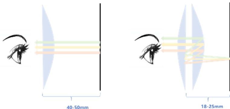
图：菲涅尔方案（左）与Pancake方案（右）对比
