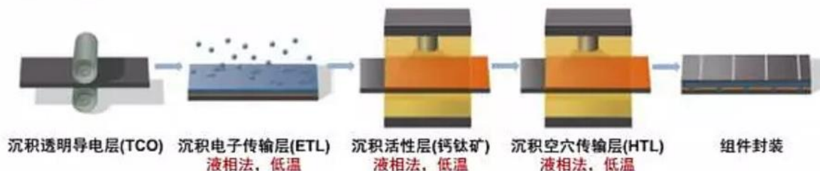
组件生产流程
