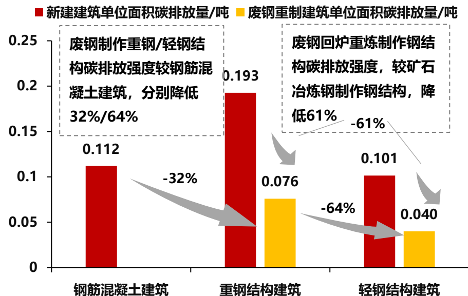
图：全寿命周期看，钢结构建筑碳排放强度
