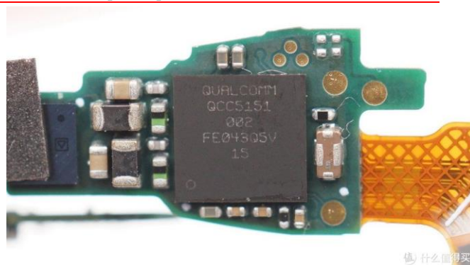
图 29 小米 Flipbuds pro 拆解 SOC 为高通 5151
