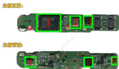
图 28 FreeBuds 4i 拆解 图中 1 为恒玄 2500Z SoC
