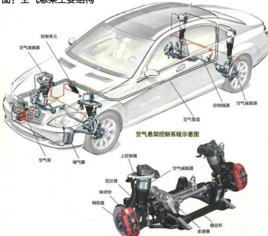
图：空气悬架主要结构
