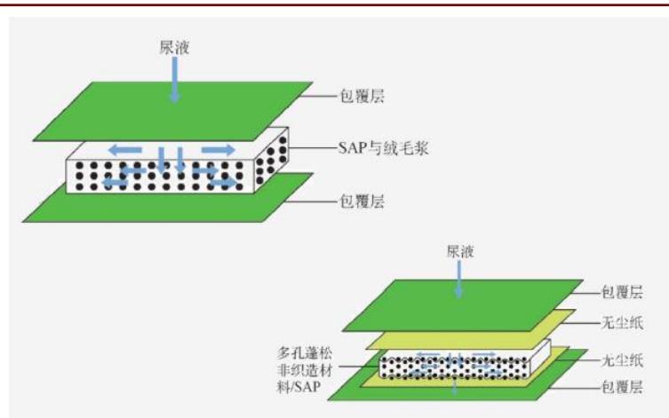
图：传统与新型吸水层结构对比
