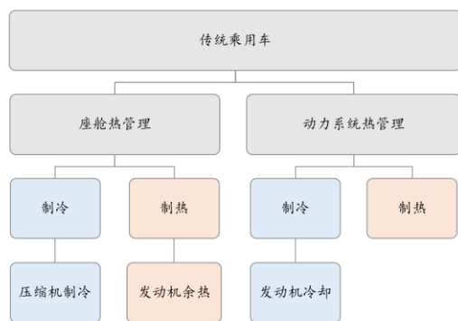
图 22、传统乘用车热管理示意图
