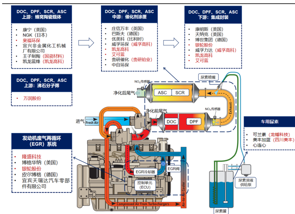
图 34、柴油机国六升级后处理零部件产业链示意图
