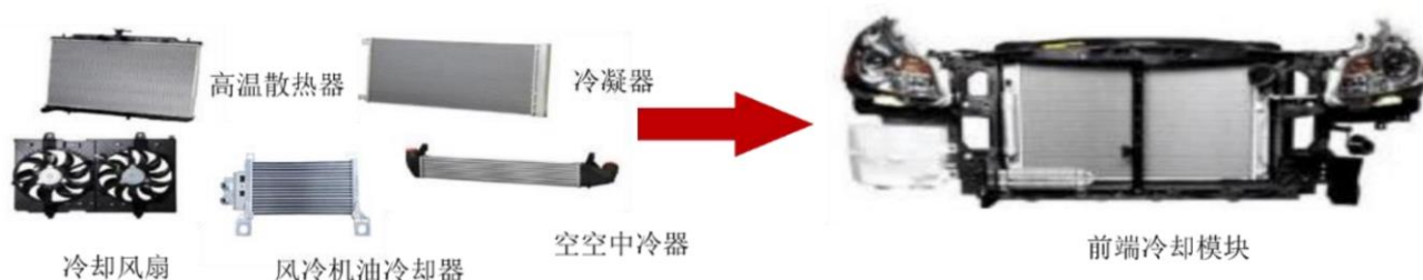
图 24、乘用车前端冷却模块的集成化
