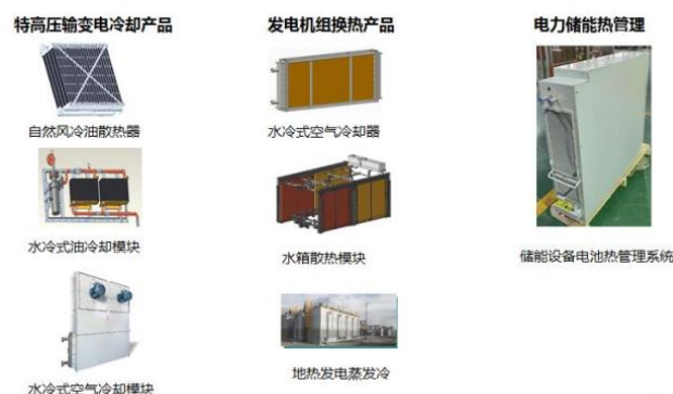
图 13、新兴领域工用/民用相关产品
