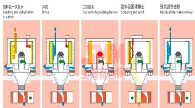
图 30：以石膏离心机为例，离心机工作流程涉及多次过滤洗涤
