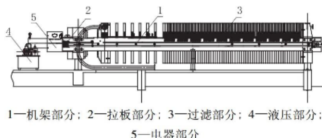
图 21：压滤机由机架、拉板、过滤、液压和电器部分组成
