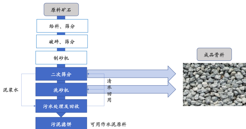
图 34：湿法制砂主要生产工艺
