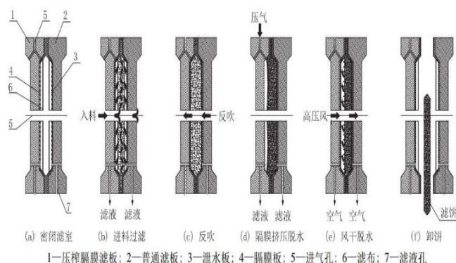
图 31：以隔膜压滤机为例，压滤机工作流程涉及连续过滤洗涤
